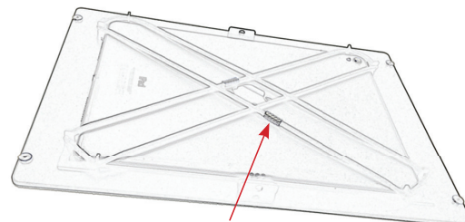
Seilklemmen
