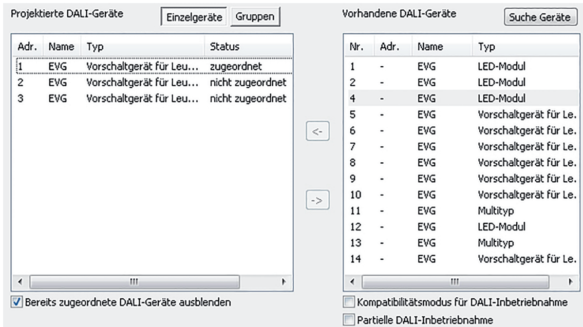
Bild 72: Betriebsgerät einem projektierten Einzelgerät zugeordnet
