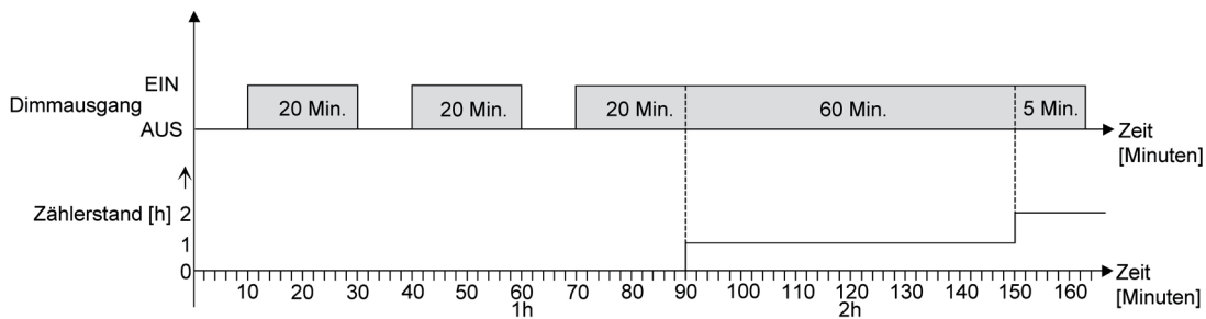
Bild 52: Funktionsweise des Betriebsstundenzählers (am Beispiel eines Vorwärtszählers)
