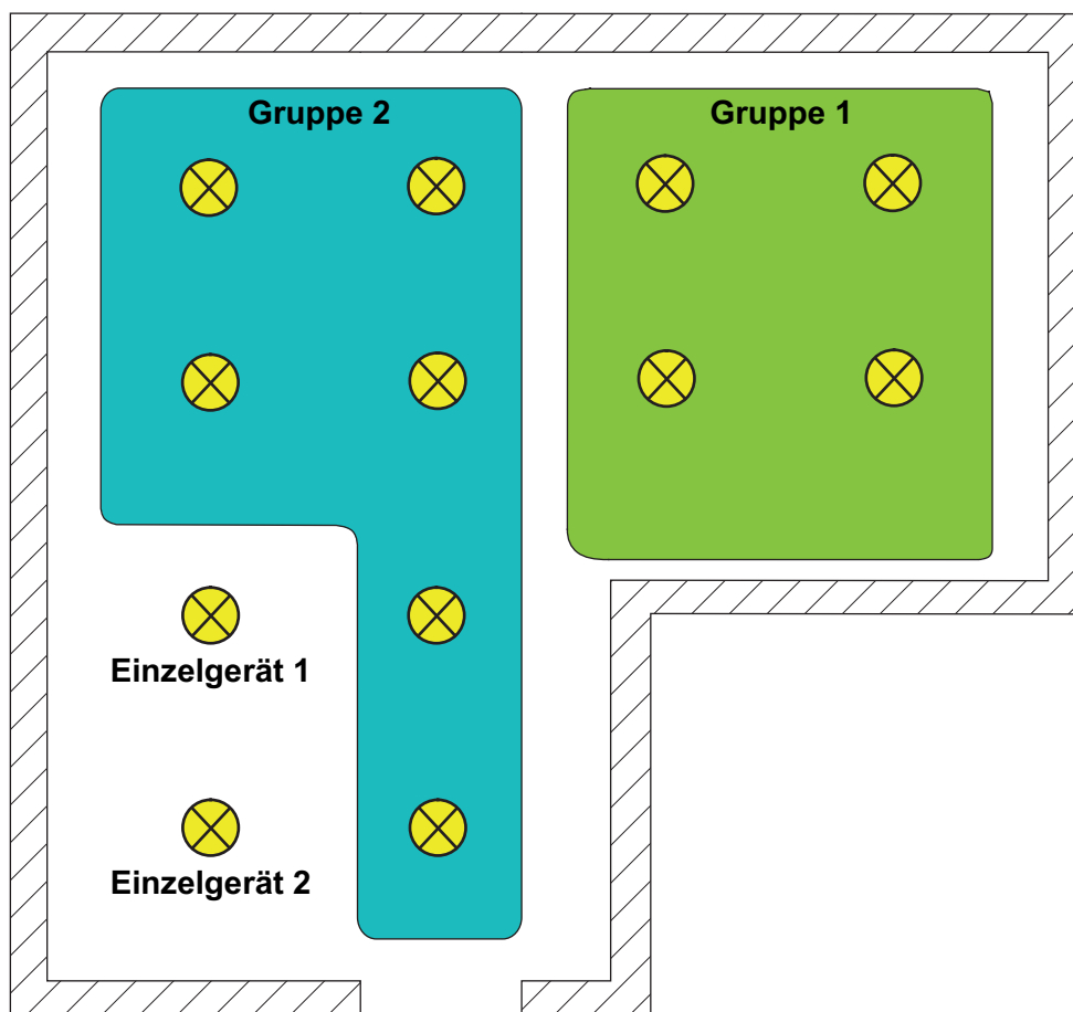
Bild 13: Beispiel einer Gruppen- und Einzelgerätsteuerung
