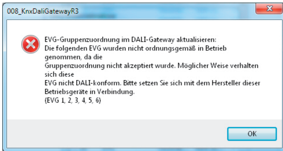
Bild 78: Fehlermeldung DALI-Gruppenzuordnung
