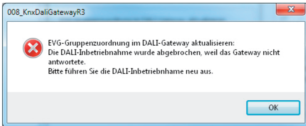
Bild 77: Fehlermeldung KNX-Kommunikationsproblem
