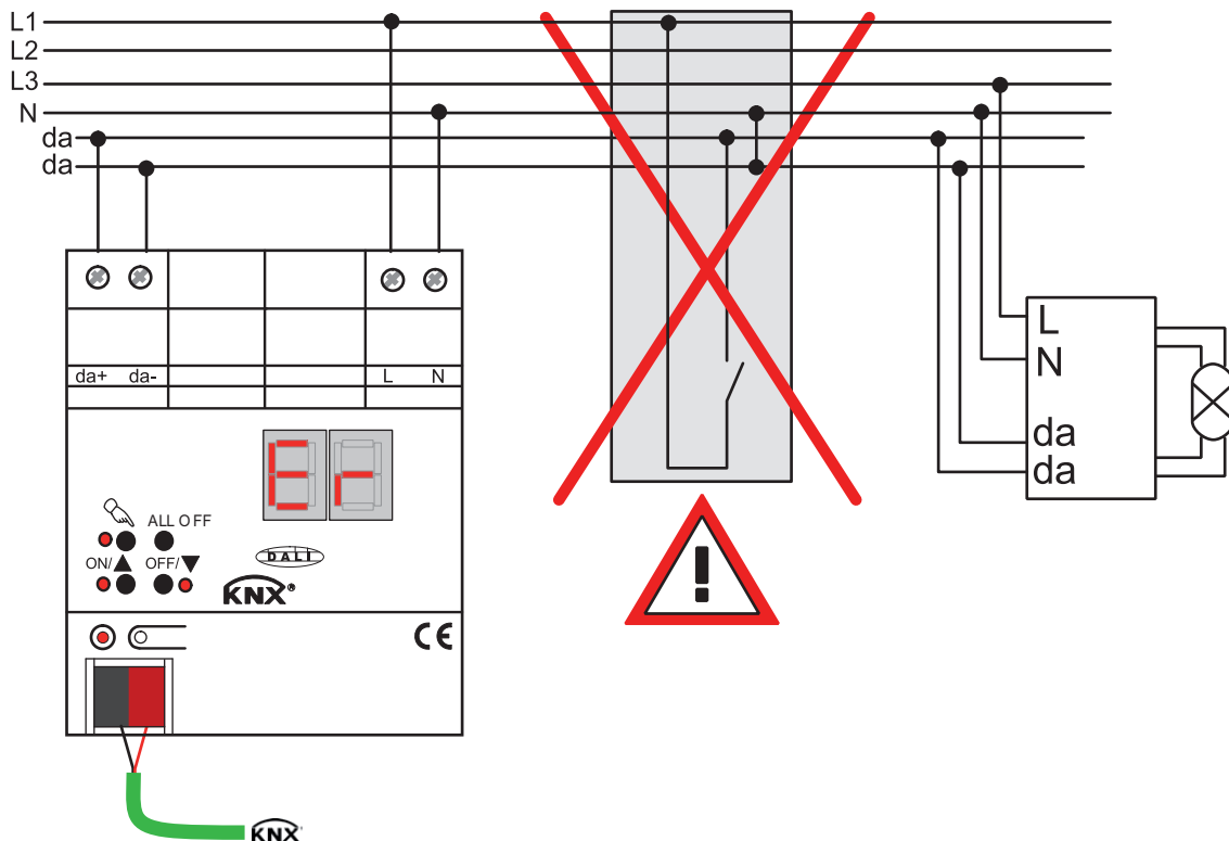
Bild 3: Andere Bedieneinrichtungen im DALI-System entfernen
