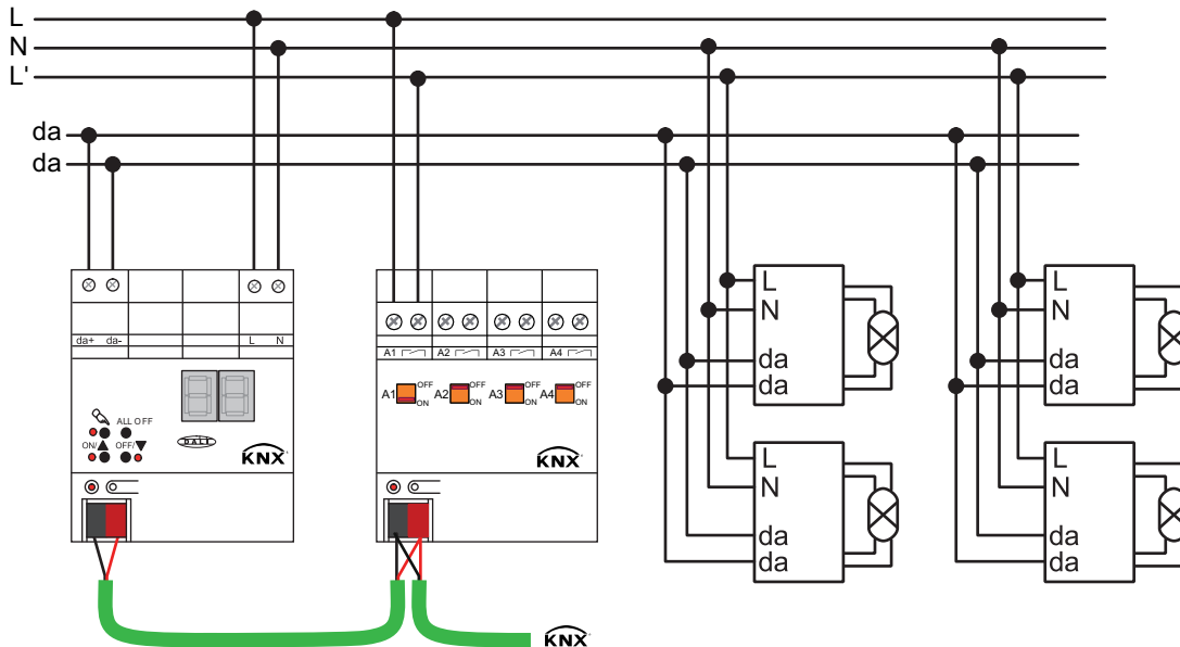
Bild 29: Beispiel eines Anschluss-Schemas zur Standby-Abschaltung durch einen KNX-Schaltaktor
