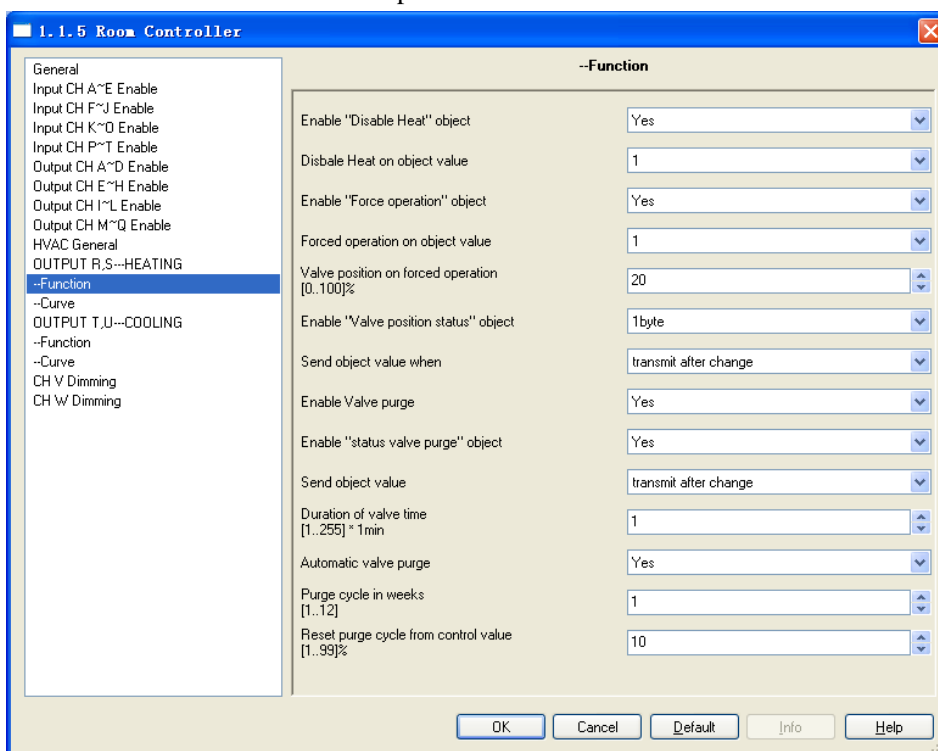
Fig. 5.36 parameter window “HEATING: Function”
