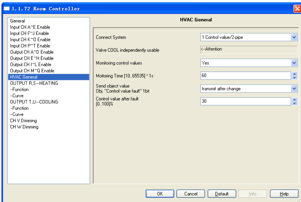
Fig. 5.34 parameter window “HVAC General”
