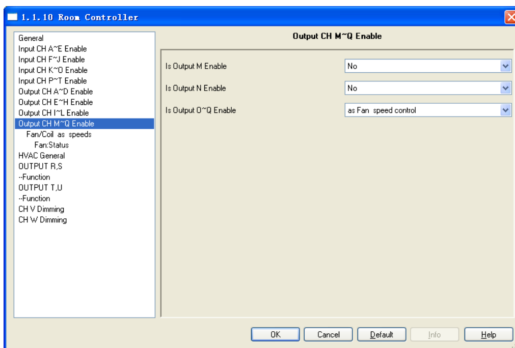
Fig. 5.26 parameter window “Output CH O~Q enable”
