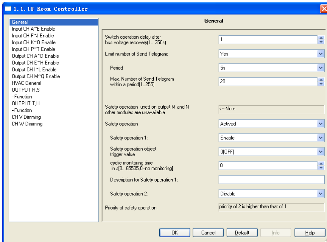
Fig. 5.1 parameter window “General”
