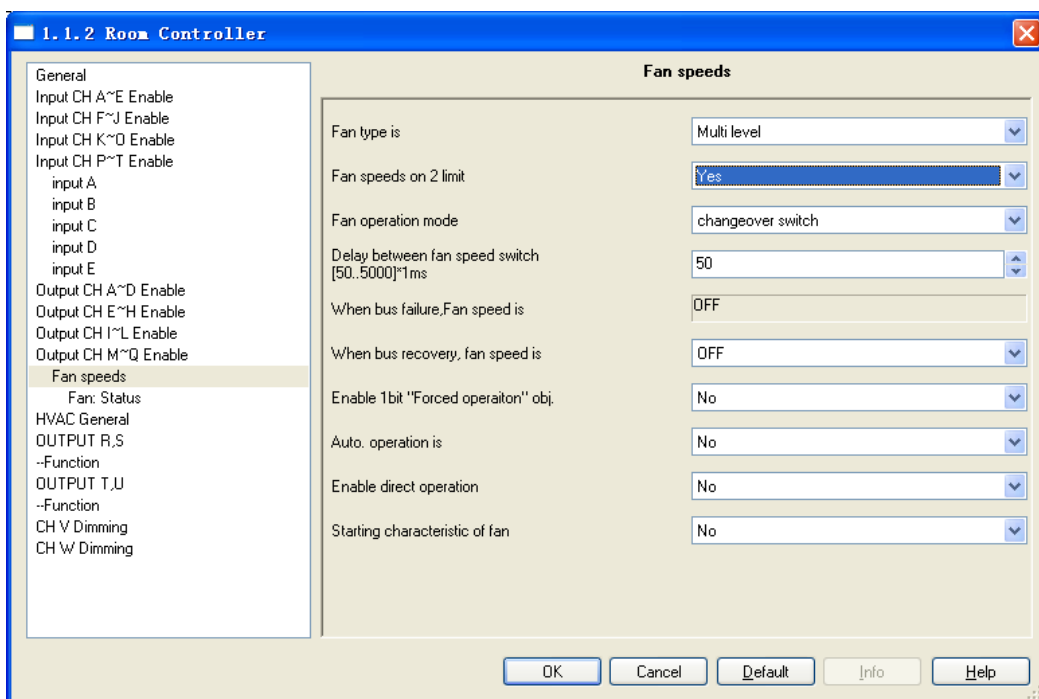
Fig. 5.30 parameter window “Fan-two level”
